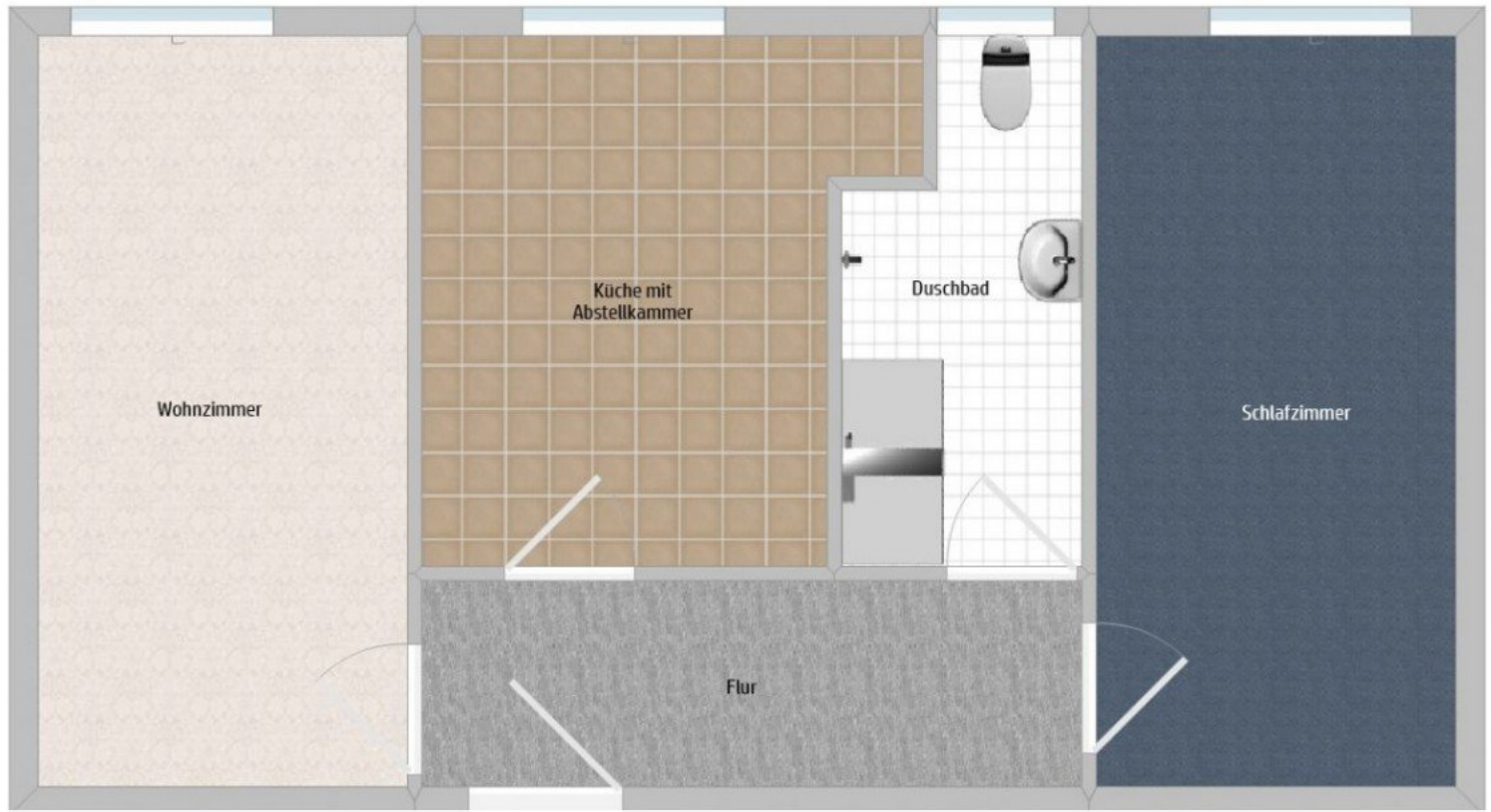
Grundriss
